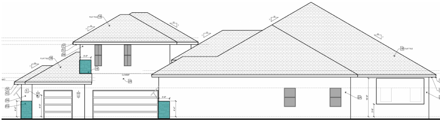
Right Elevation
